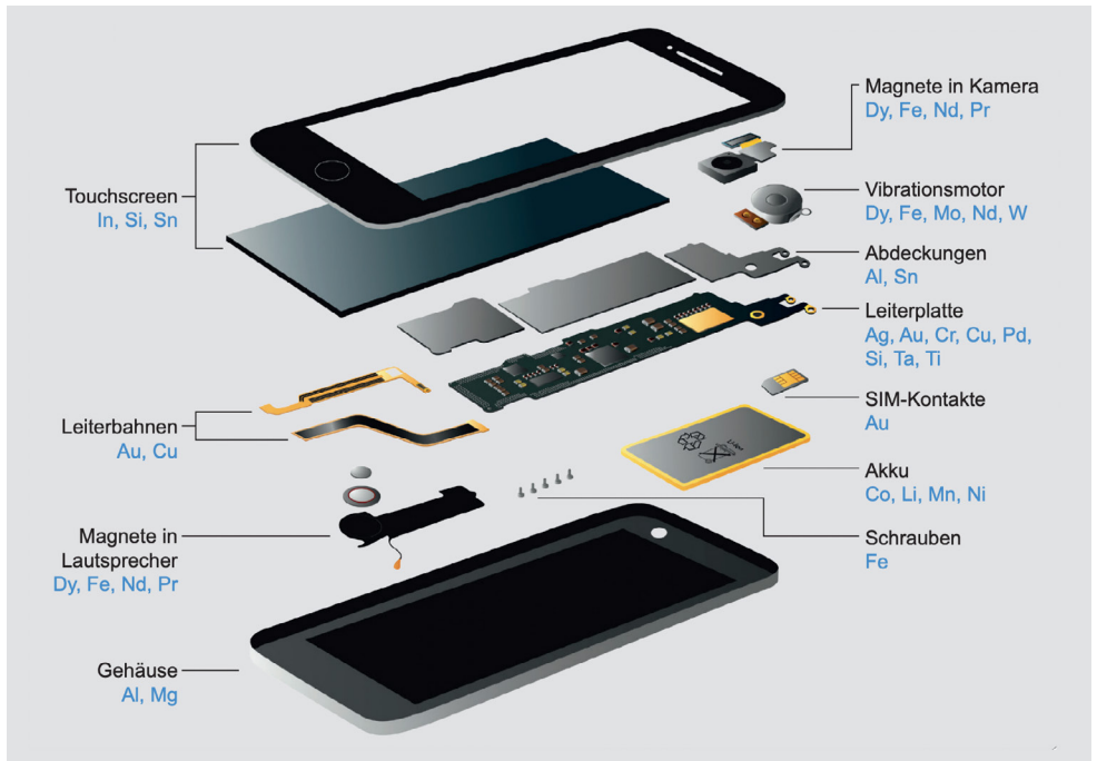
Abb. 3: Zerlegtes Smartphone und darin vorkommende Metalle (© BGR/PrinzMayer)
